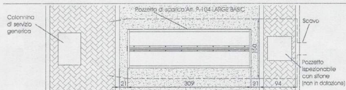
Particolare costruttivo pozzetto scarico camper
